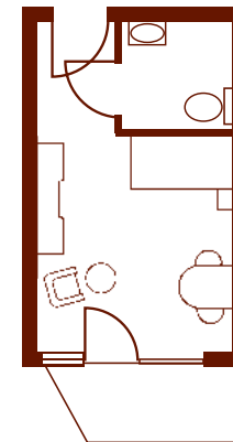
Grundriss-Beispiel eines Einzelzimmers
